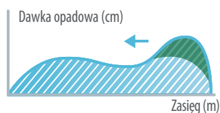
Profil rozprowadzania z niskim ciśnieniem
