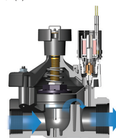
Przekrój zaworu PEB
