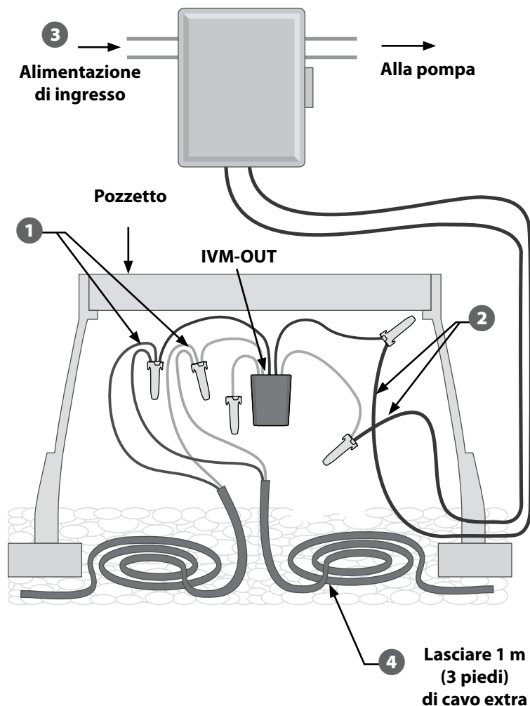
Collegamento tipico del relè avvio pompa IVM-OUT
