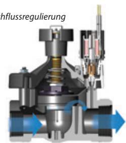
PEB Schnittdarstellung
